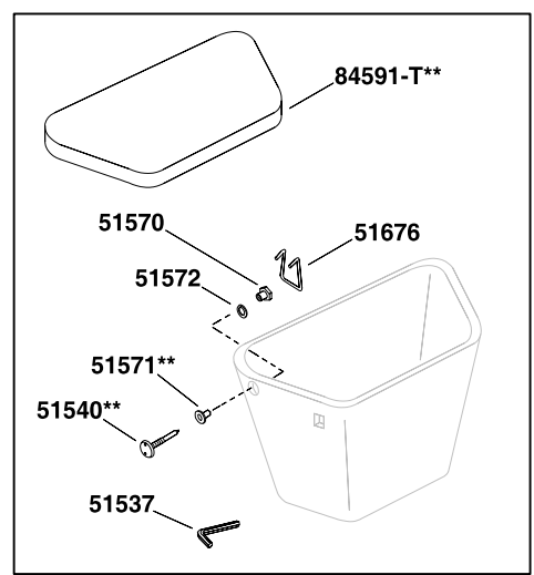
Tank Lock Option (one side shown) Option verrouillage réservoir (un côté illustré) Opción de seguros para el tanque (se ilustra un lado)
